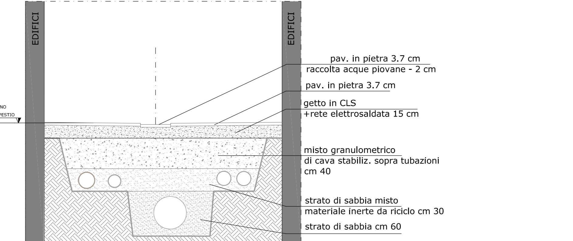
SEZIONE TIPO
